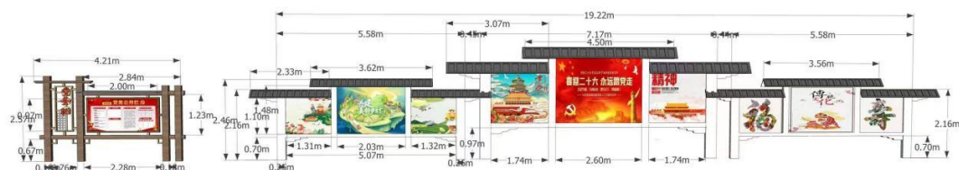
长廊立面尺寸图：
